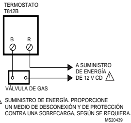
Fig. 6. T812B en aplicación de 12 V cd.
