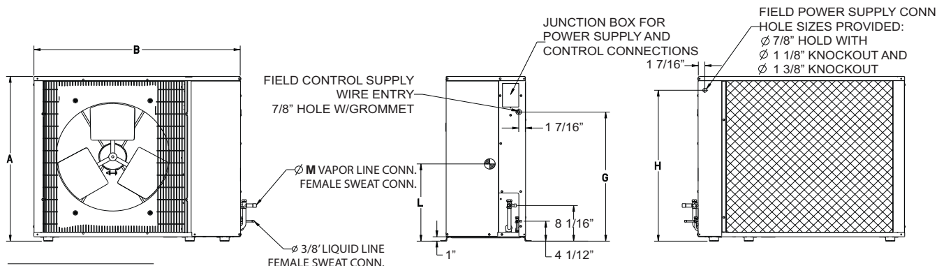
Fig. 3 — Dimensions
