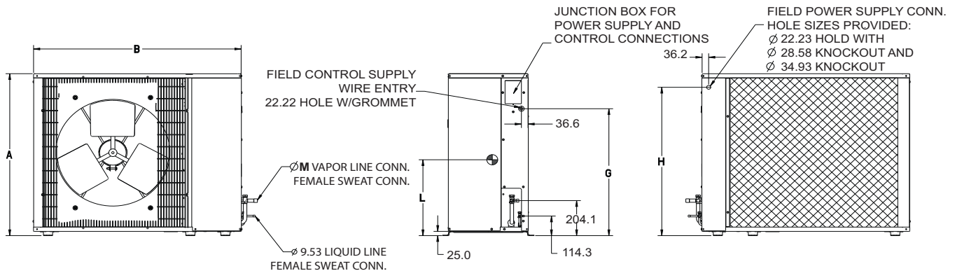
Fig. 5 — Dimensions
