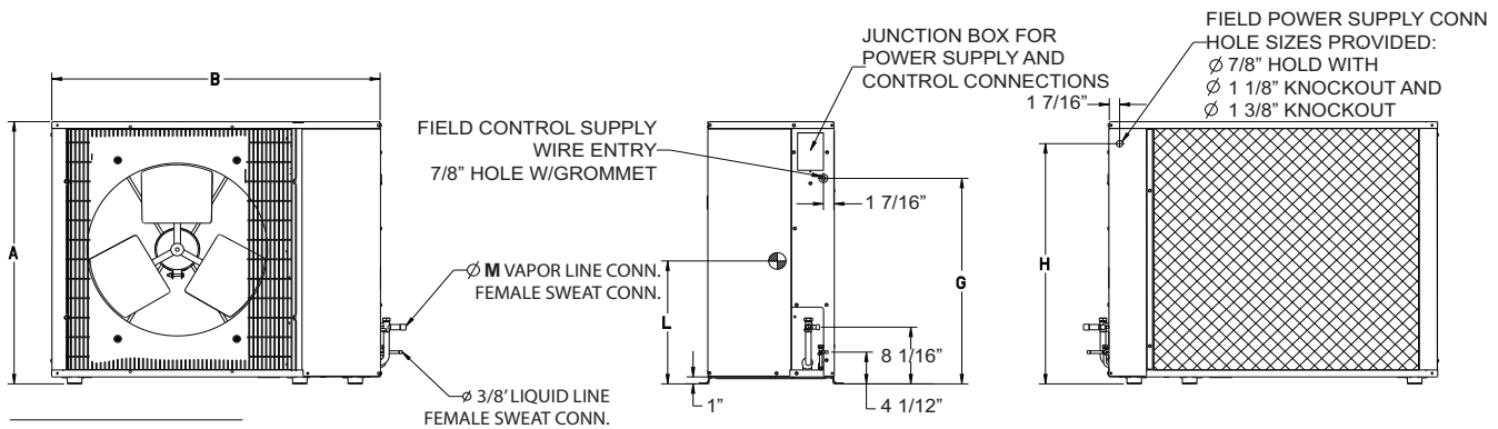
Fig. 3 — Dimensions
