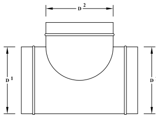
SP6271 90° TEE
