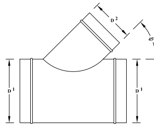
SP6276 45° LATERAL
